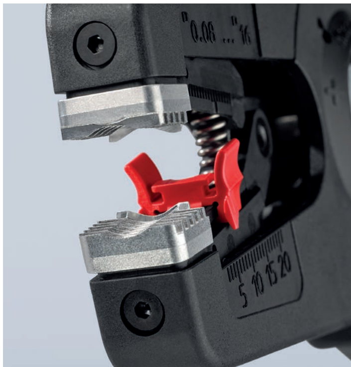
Le ganasce semicirculari con profilo a pettine per una migliore presa tengono praticamente qualsiasi isolante in modo sicuro
