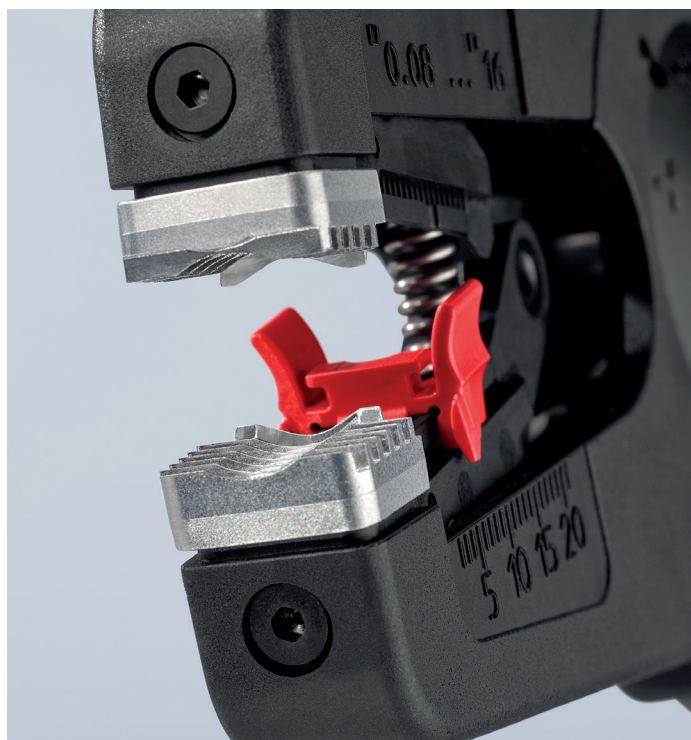
Halvrunde holdekæber med kamprofil sikrer bedre greb og holder alle isoleringsmaterialer sikkert fast
